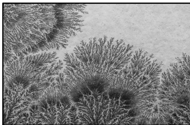
איור 41: צילום של המינרל פירולוזיט המופיע בצורה דנטריתית (קליין, 2015, עמ' 144)
